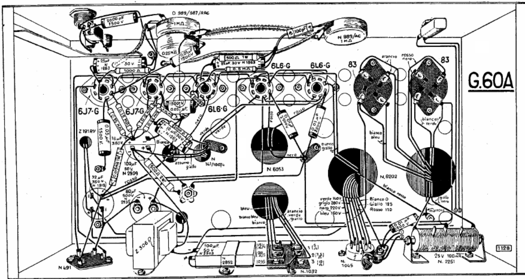
Lo schema costruttivo del G-60 A
